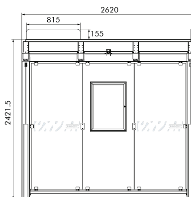
Réf. 529411
