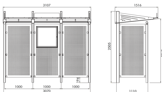
Réf. 529435 + 209115
