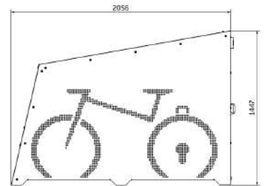
■ Réf. 529450 + 529454 + 529455
