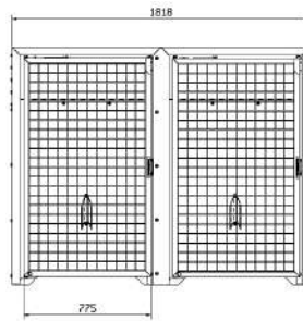
■ Réf. 529450 + 529454 + 529455
