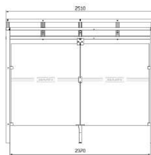
■ Réf. 529170 + 209147
